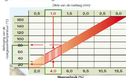
Figuur 2: Ketelvervuiling en meerverbruik.
