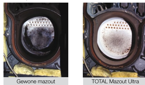
Figuur 1: Binnenkant van een ketel na verbrandingsproeven.
